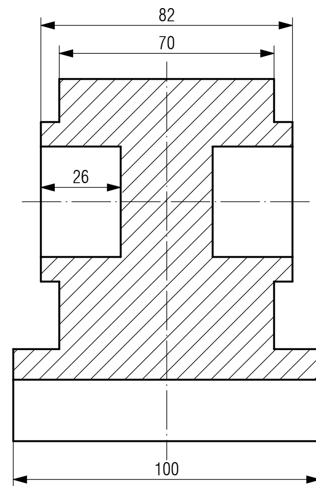
CORTE A-A
